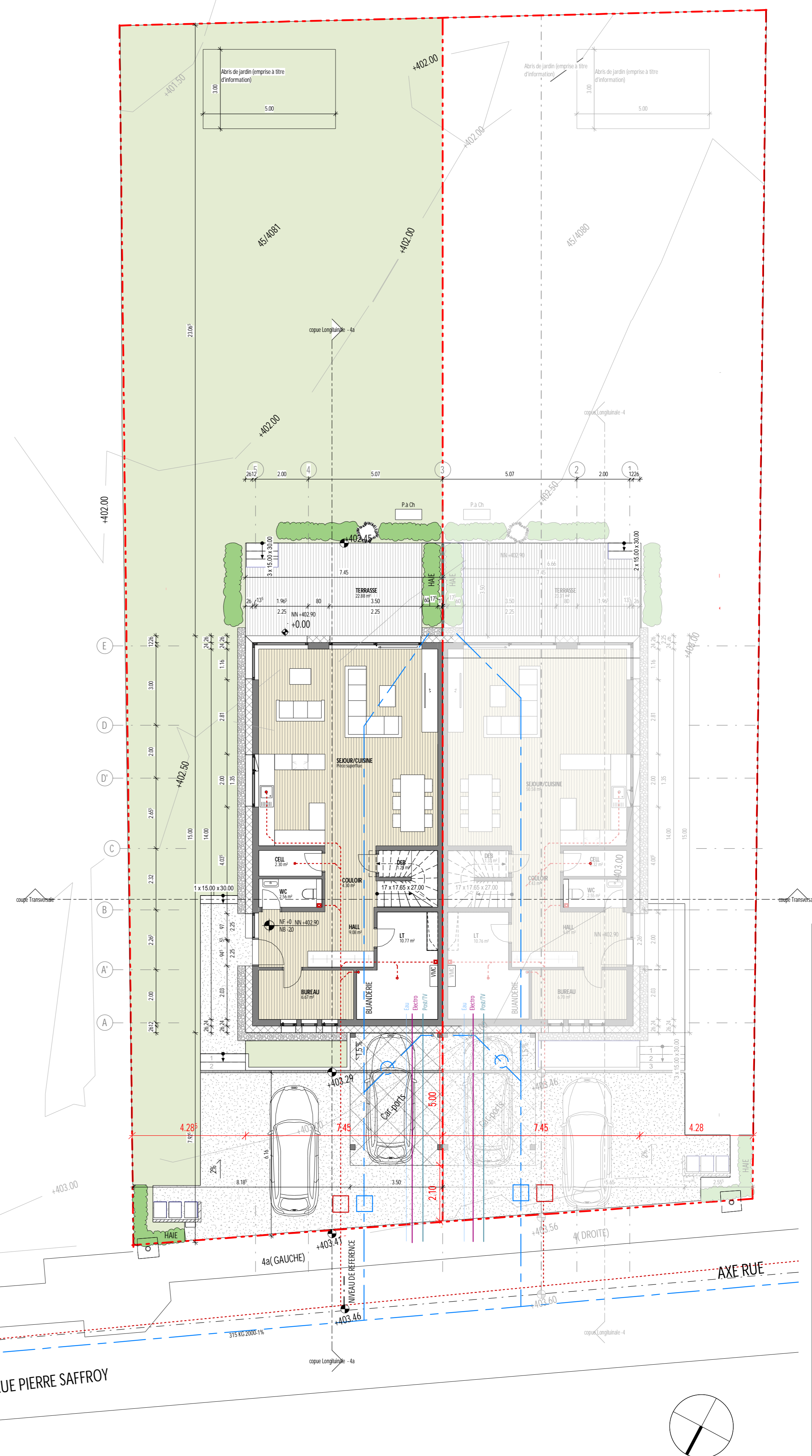
PLAN DU REZ-DE-CHAUSSEE M: 1/100
