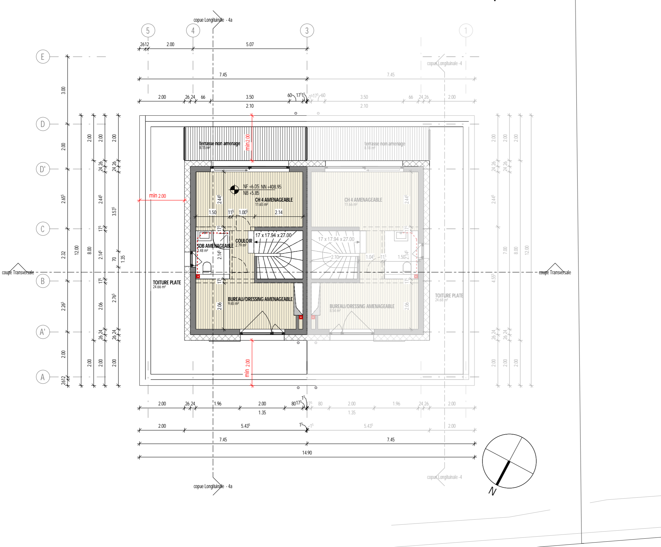
PLAN DU 1er ETAGE M: 1/100
