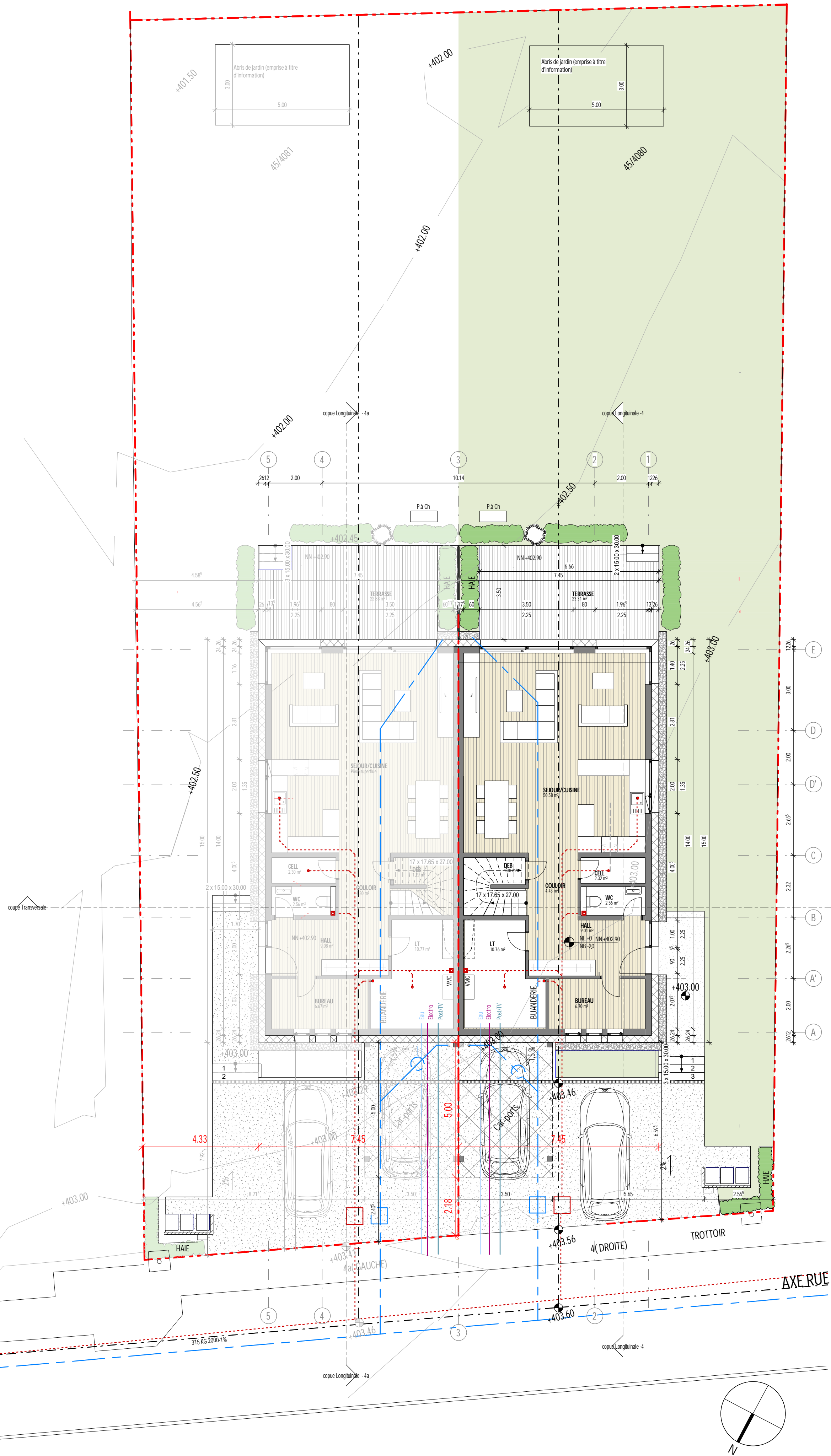
PLAN DU REZ-DE-CHAUSSEE M: 1/100
