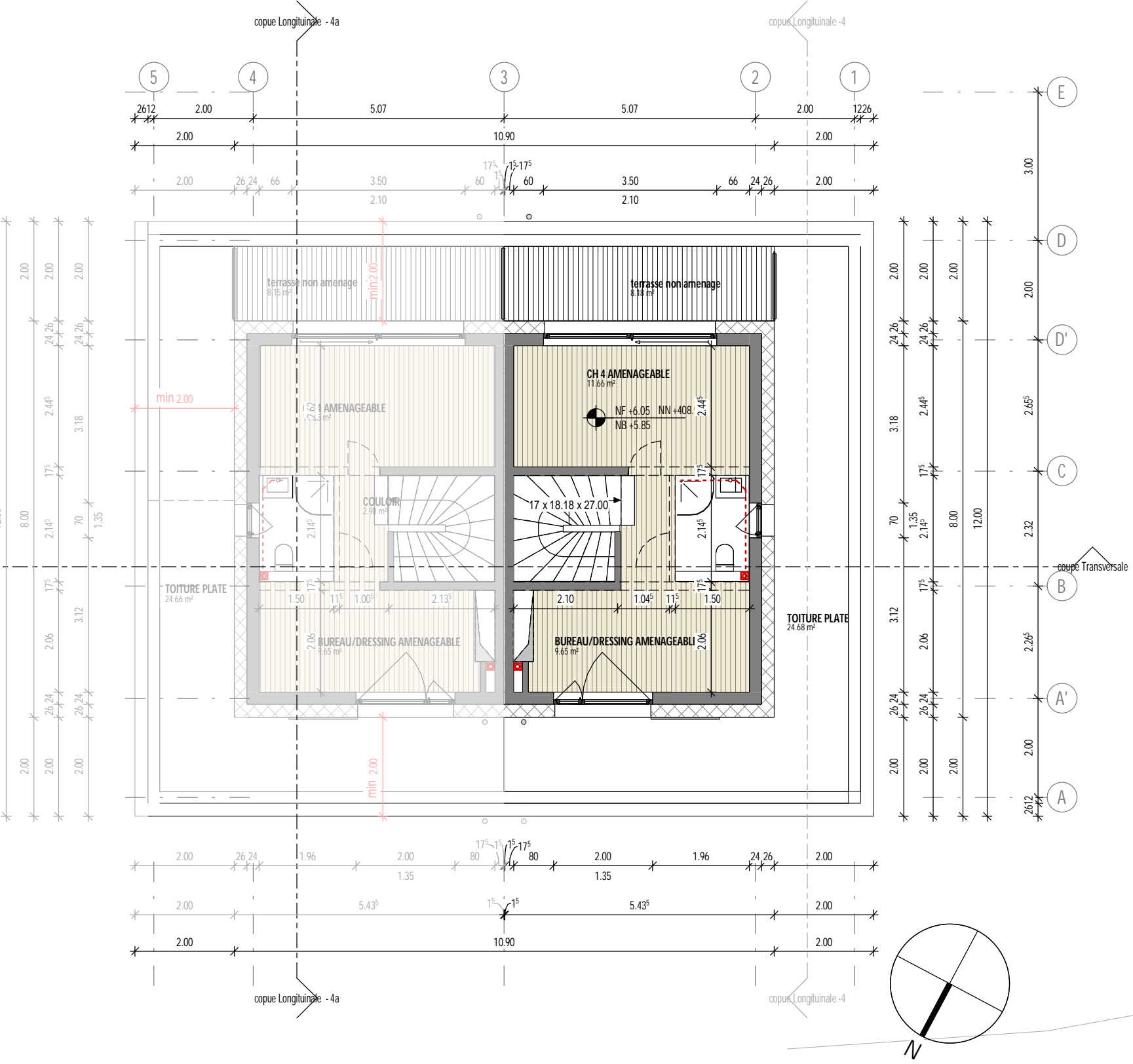
PLAN DU 1er ETAGE M: 1/100
