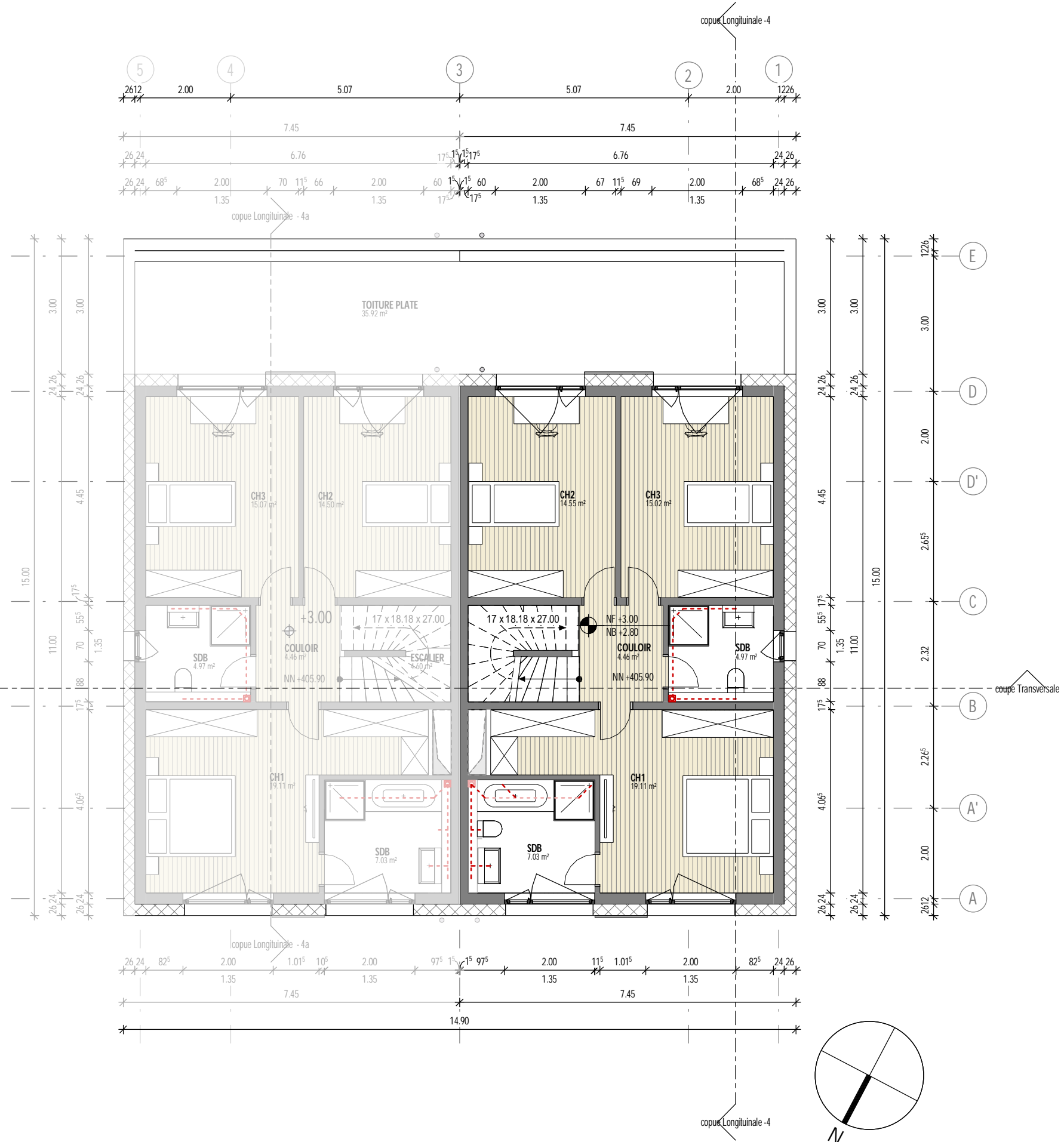
PLAN DU 1er ETAGE M: 1/100
